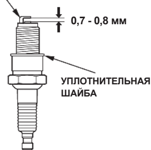
БОКОВОЙ ЭЛЕКТРОД
