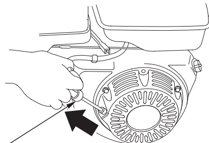
РУЧКА СТАРТЕРА
