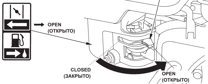
РЫЧАГ ВОЗДУШНОЙ ЗАСЛОНКИ
