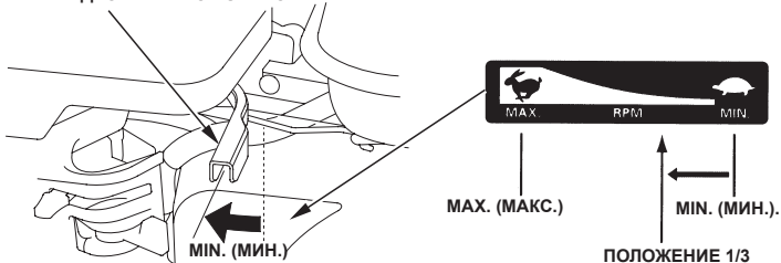
РЫЧАГ ДРОССЕЛЬНОЙ ЗАСЛОНКИ
