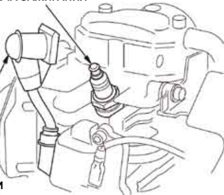
СВЕЧА ЗАЖИГАНИЯ
