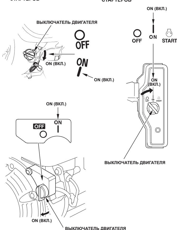
ТИПЫ ЭЛЕКТРИЧЕСКИХ СТАРТЕРОВ
