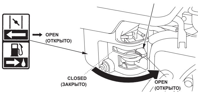
РЫЧАГ ВОЗДУШНОЙ ЗАСЛОНКИ
