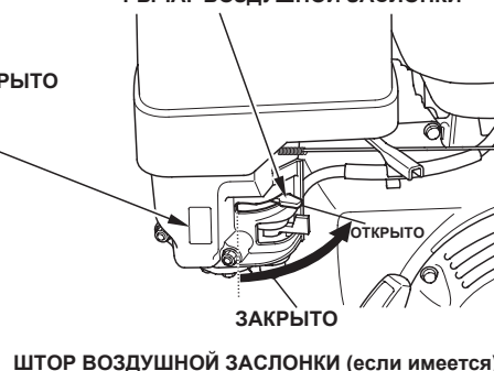
ШТОР ВОЗДУШНОЙ ЗАСЛОНКИ (если имеется)
